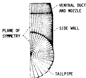
(b) END VIEW (yz-PLANE).
